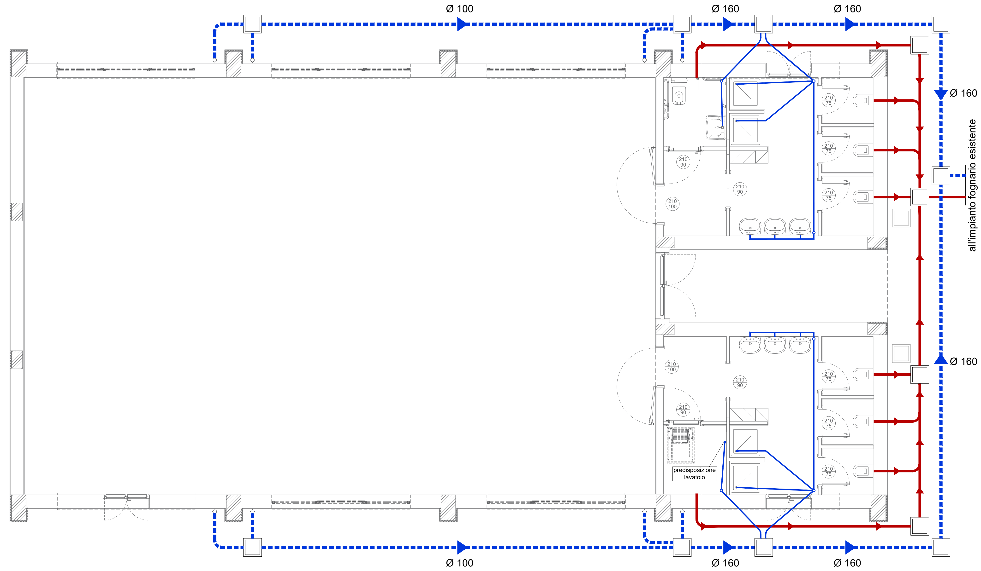
Pianta quota 0.15 metri - Progetto scala 1:50
